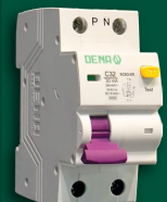
محافظ جان 6000 (RCBO)
